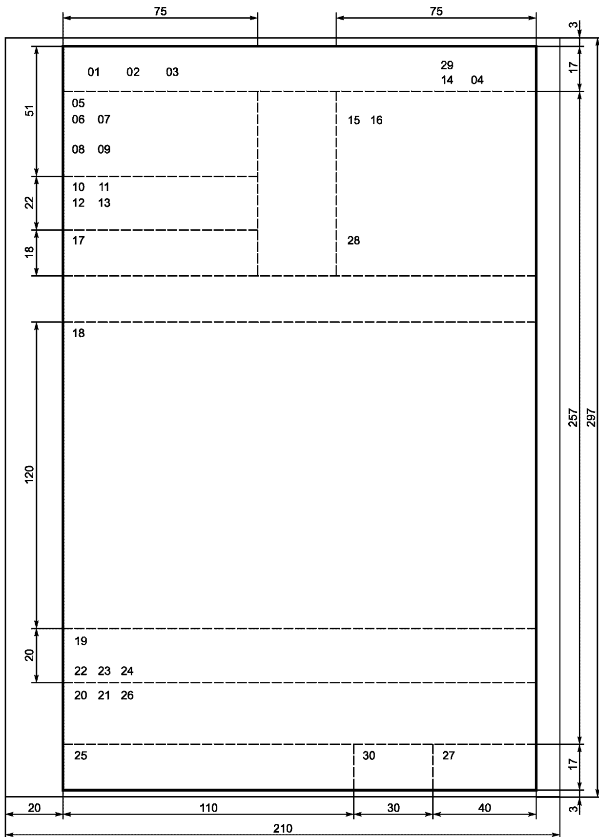
Рисунок А.1 – расположение реквизитов и границ зон на формате А4 углового бланка
