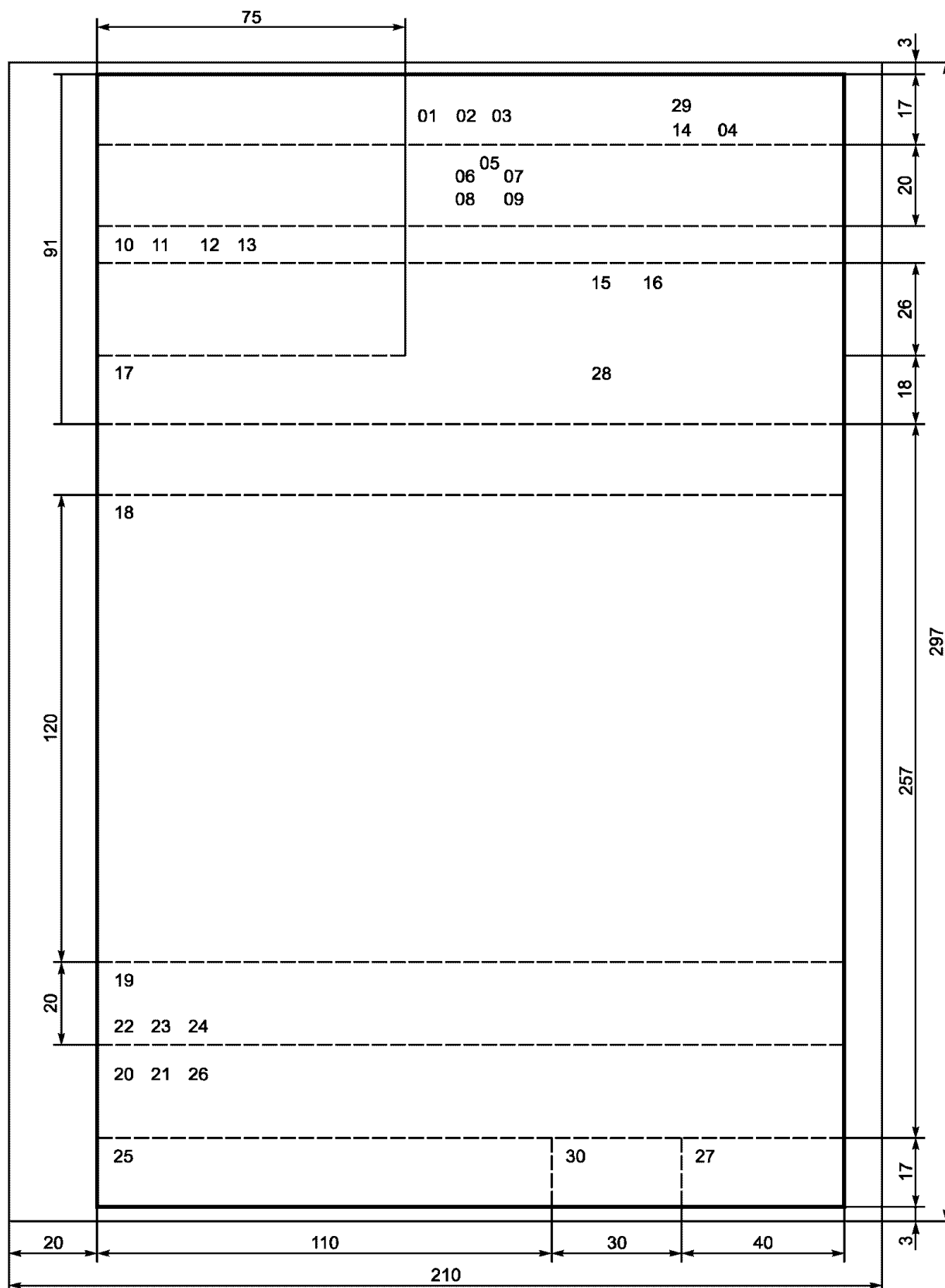
Рисунок А.1 – расположение реквизитов и границ зон на формате А4 продольного бланка
